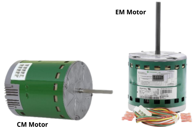
CM Motor
